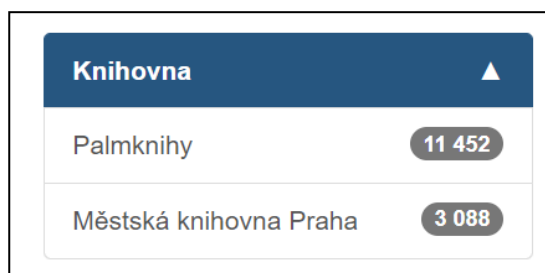
Obrázek 3: Filtr e-knihy
